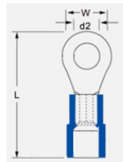
Crimp-Ringkabelschuh
