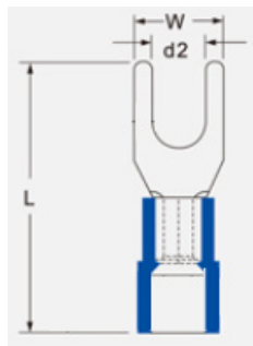
Crimp-Gabelkabelschuh
