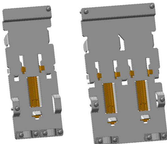
Adapter für DIN-Schienenmontage für FSAA/FSAB/FSA
